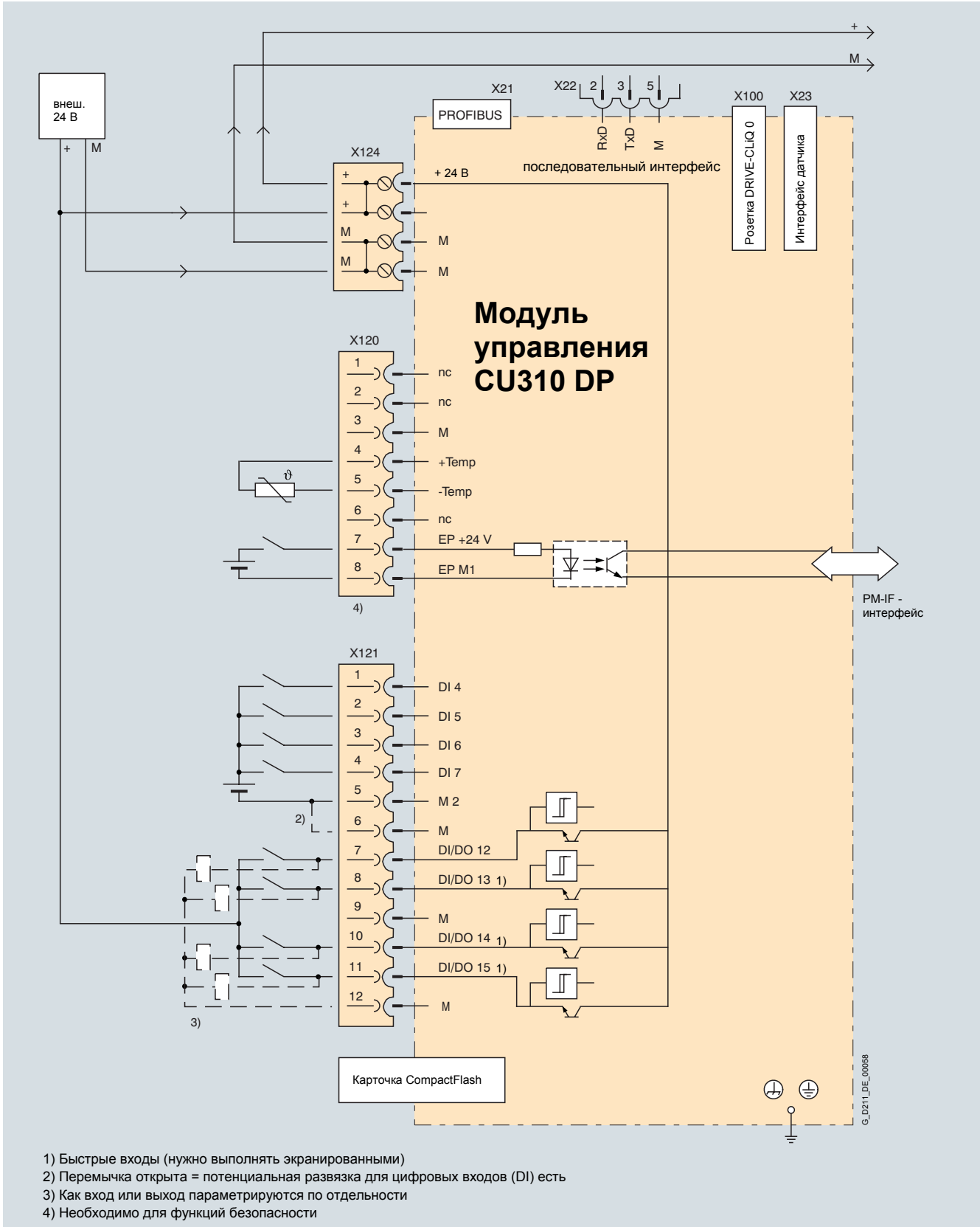
Пример подключения модуля управления CU310 DP
