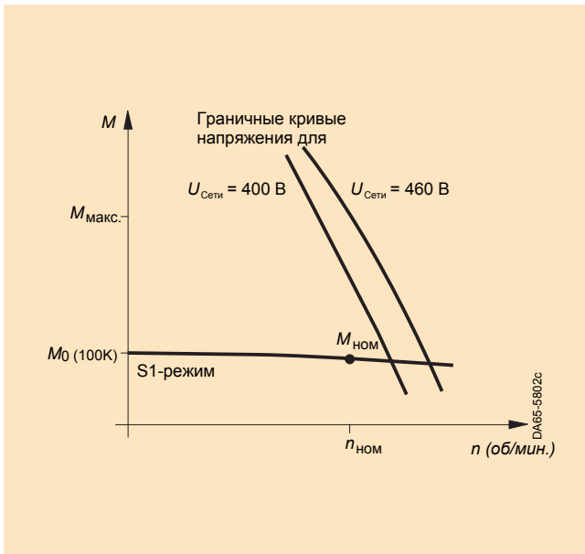
Характеристика крутящий момент / скорость
