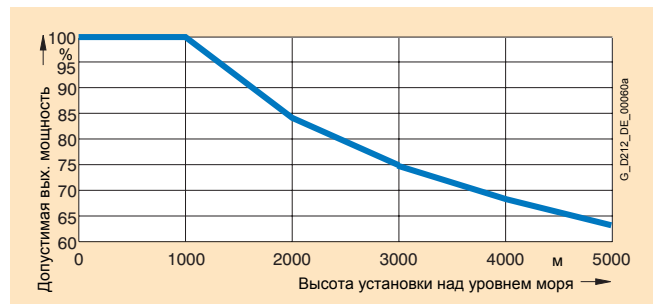
Выходная мощность в зависимости от высоты установки
