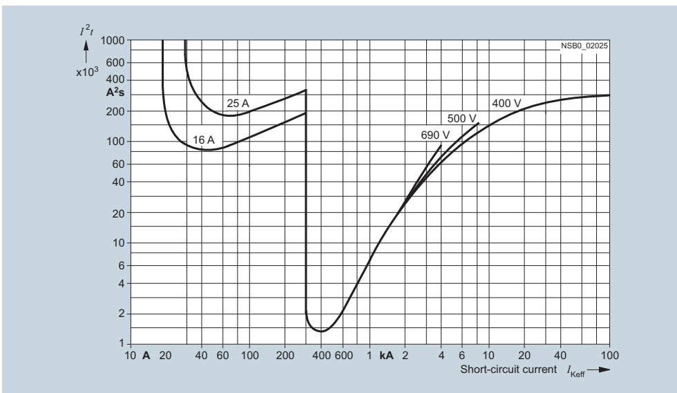
Характеристика I²t для 3VS1600-0MN00
