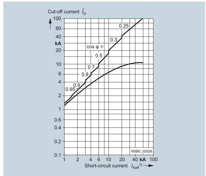
Характеристика токоограничения для 3VS1600-0MN00
