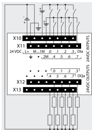
6ES7 223-1BH32-0XB0*
