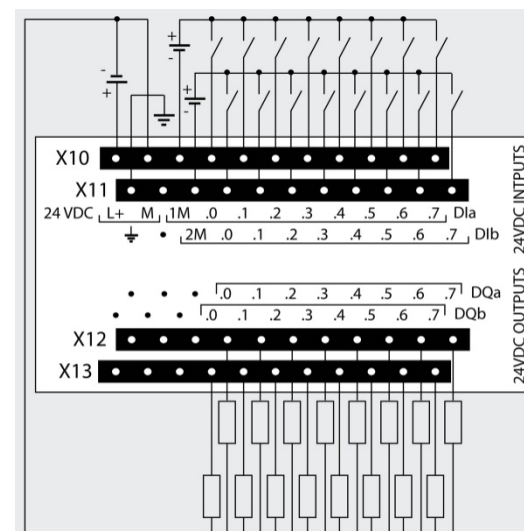
6ES7 223-1BL32-0XB0*
