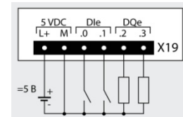
6ES7 223-3AD30-0XB0
