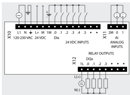
6ES7 211-1BE40-0XB0
